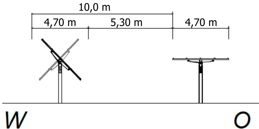
Abbildung 3: Vertikalschnitt - Quelle: Auftraggeber
